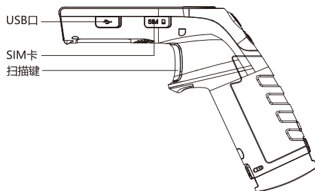
图2 左视图
