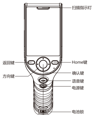
图1 正面视图
