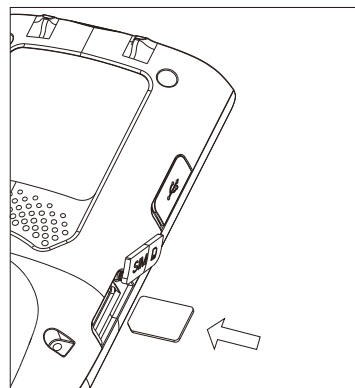
Рис. 4 Установка SIM-карты
