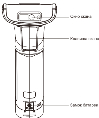
Рис. 3 Передний вид
