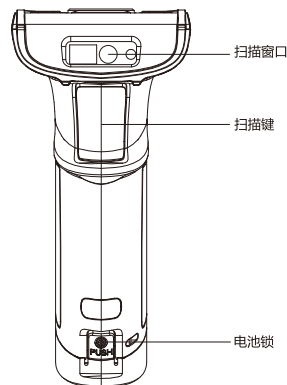
图3 前视图
